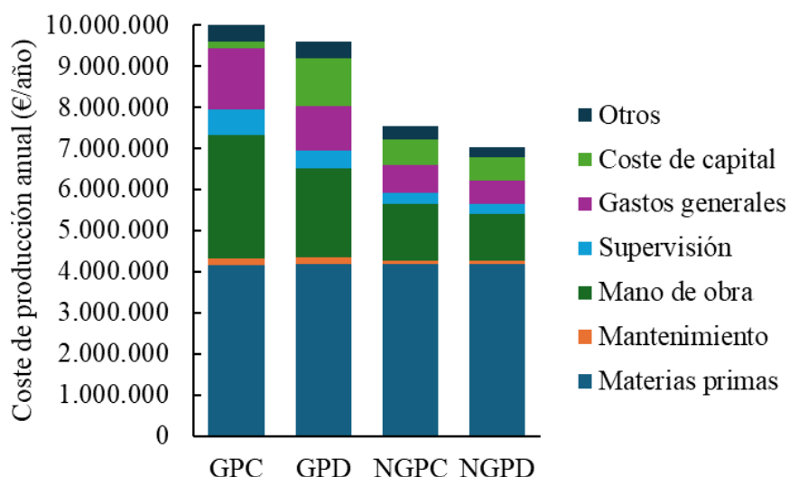
Figura 28. Distribución del coste de producción anual para cada escenario.
