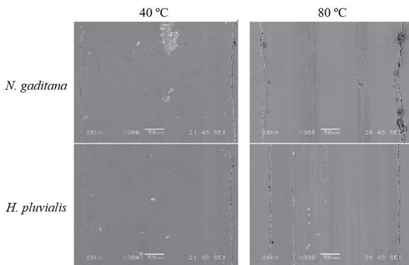
Figura 15. Imágenes del SEM de las superficies del disco tras los ensayos de deslizamiento alternativo para los FAMES derivados de N. gaditana y H. pluvialis .
