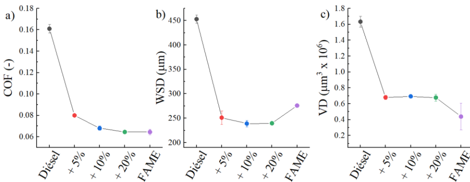
Figura 25. Efecto de la adición de FAME derivado de H. pluvialis en un diésel puro: a) COF medio; b) desgaste en la bola WSD; c) volumen de desgaste en el disco VD.
